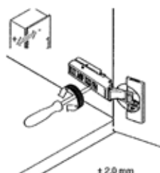
Sideveisregulering
